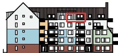
Fasad mot norr
